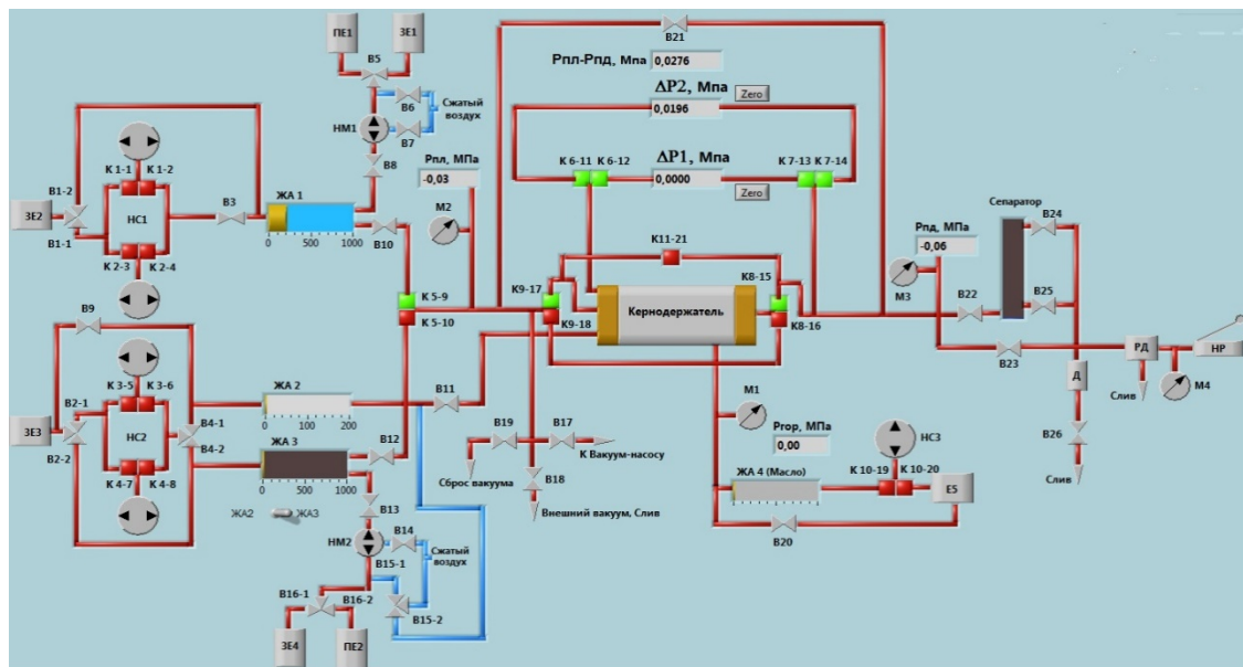
Рис. 27. Схема установки ПЛАСТ.АТМ-10.
