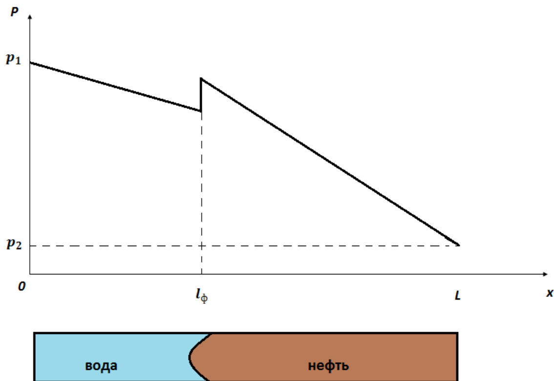
Рис. 13. Распределение давления в капилляре при вытеснении нефти водой.
