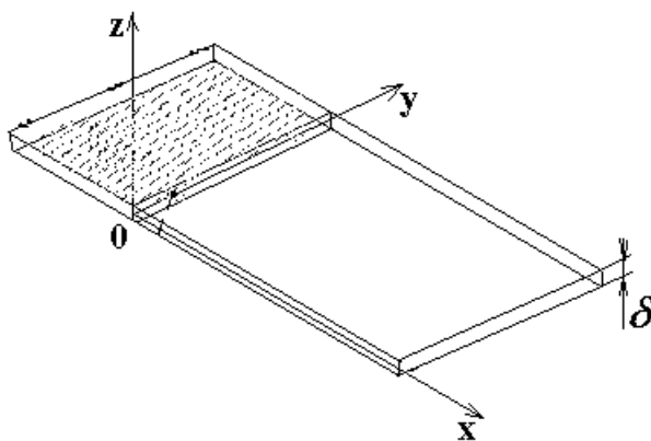
Рис. 18. Ячейка Хеле-Шоу.
