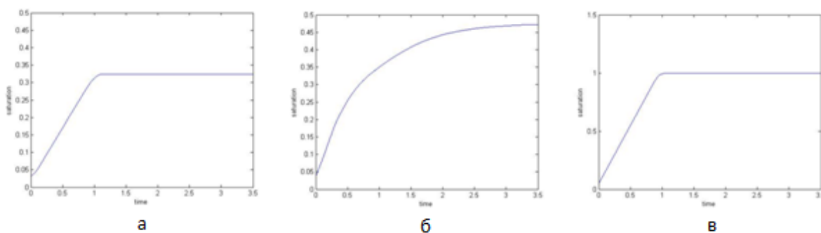
Рис. 26. Зависимость насыщенности вытесняющей жидкости от времени.
