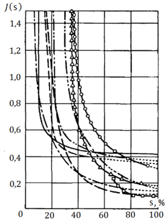
Рис. 14. Функции Леверетта.
