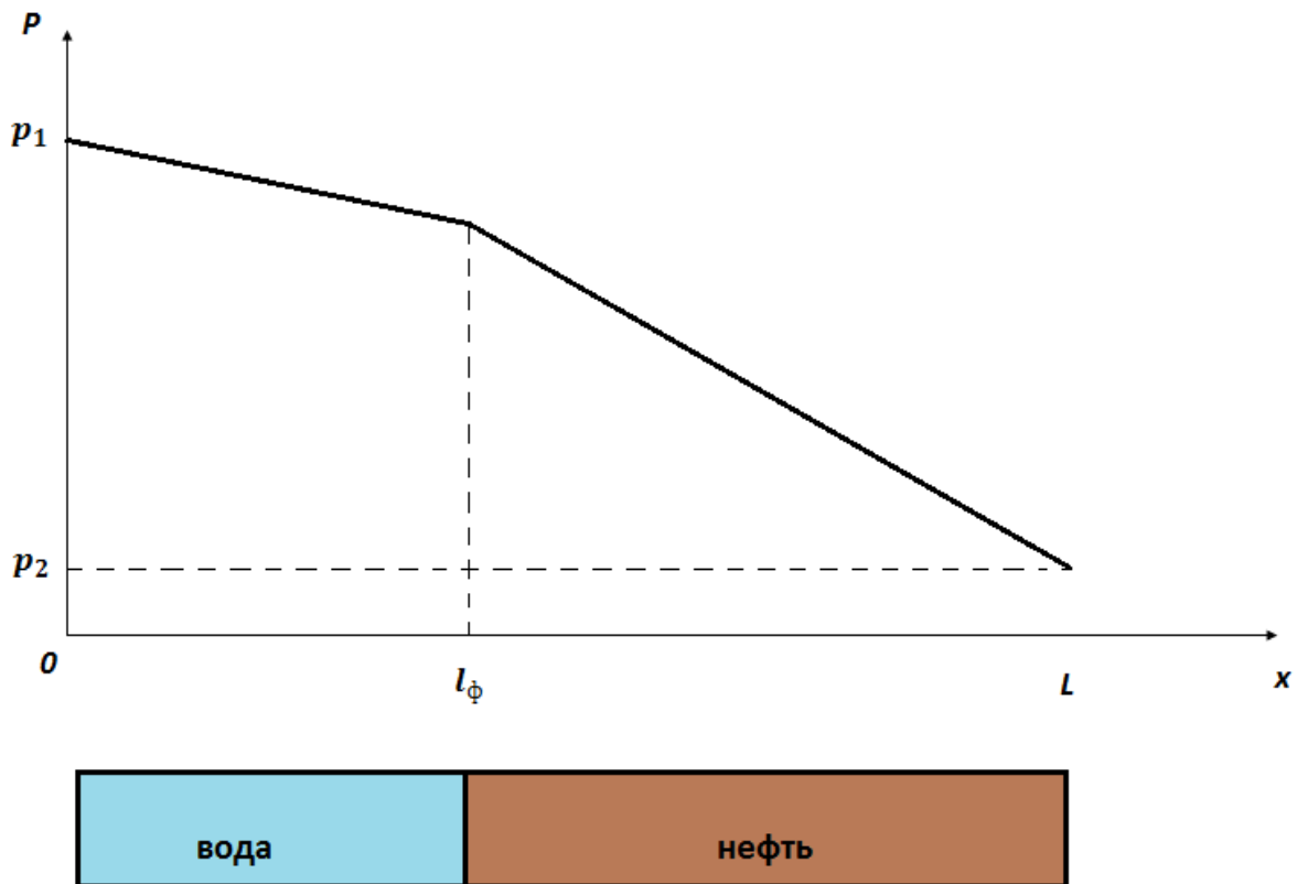
Рис. 9. Распределение давления при поршневом вытеснении.
